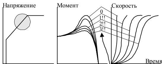
Кривые разгона 0, 1, 2, 3 для насоса
