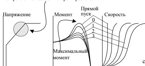
Управление насосом во время разгона
